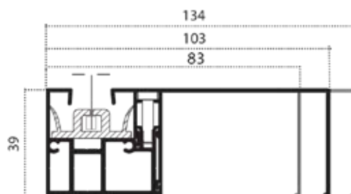
ΚΡΥΦΟΣ ΟΔΗΓΟΣ (ΟΔΗΓΟΣ ΜΕ ΕΞΟΧΗ) HIDDEN GUIDE
