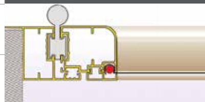
ΠΡΟΦΙΛ "Z" ΚΑΤΟΠΙΝ ΠΑΡΑΓΓΕΛΙΑΣ FRAME PROFILE "Z" UPON REQUEST
